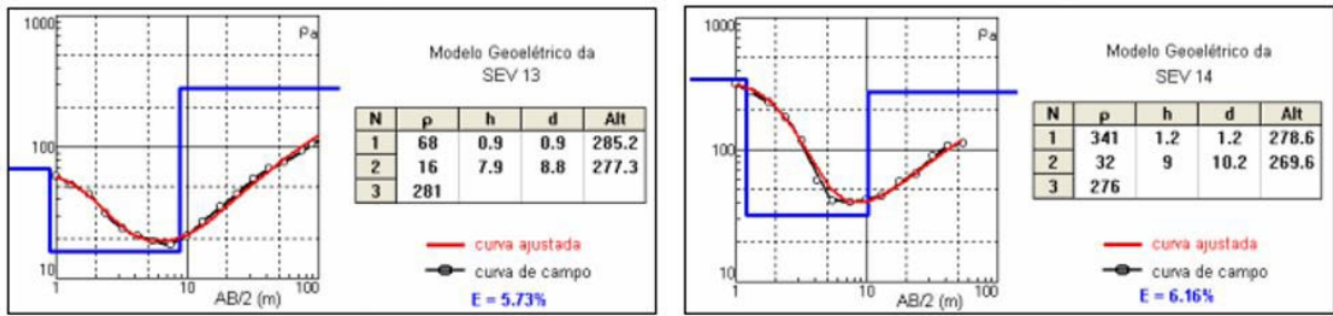
Figura 17 – Modelo geoeétrico das SEVs 13 e 14.
