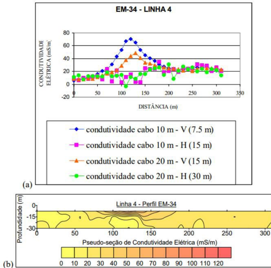
Figura 33 – Perfil de caminhamento eletromagnético da Linha 4 em a) condutividade em função da distância e em b) isovalores da condutividade com a profundidade.
