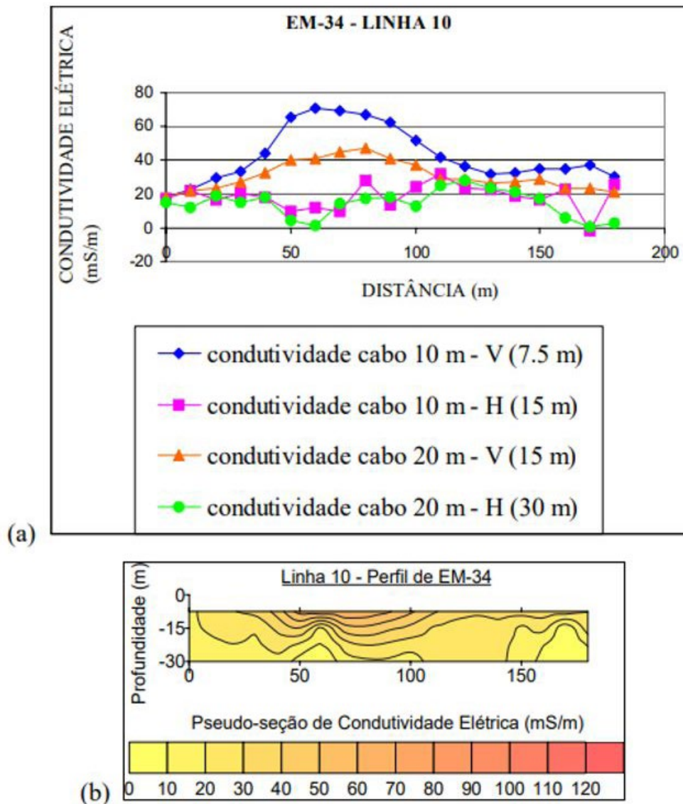
Figura 37 – Perfil de caminhamento eletromagnético da Linha 10 em a) condutividade em função da distância e em b) isovalores da condutividade com a profundidade.
