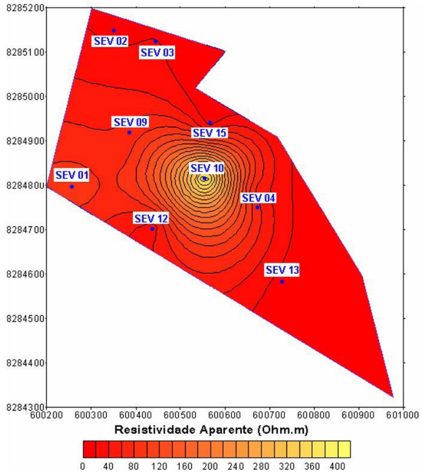
Figura 23 – Mapa de resistividade para a cota 280 metros.
