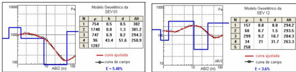
Figura 14 – Modelo geoeétrico das SEVs 01 e 12.
