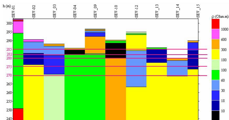
Figura 20 – Seções de resistividade do modelo geológico das SEVs com os níveis para elaboração dos mapas de resistividade.
