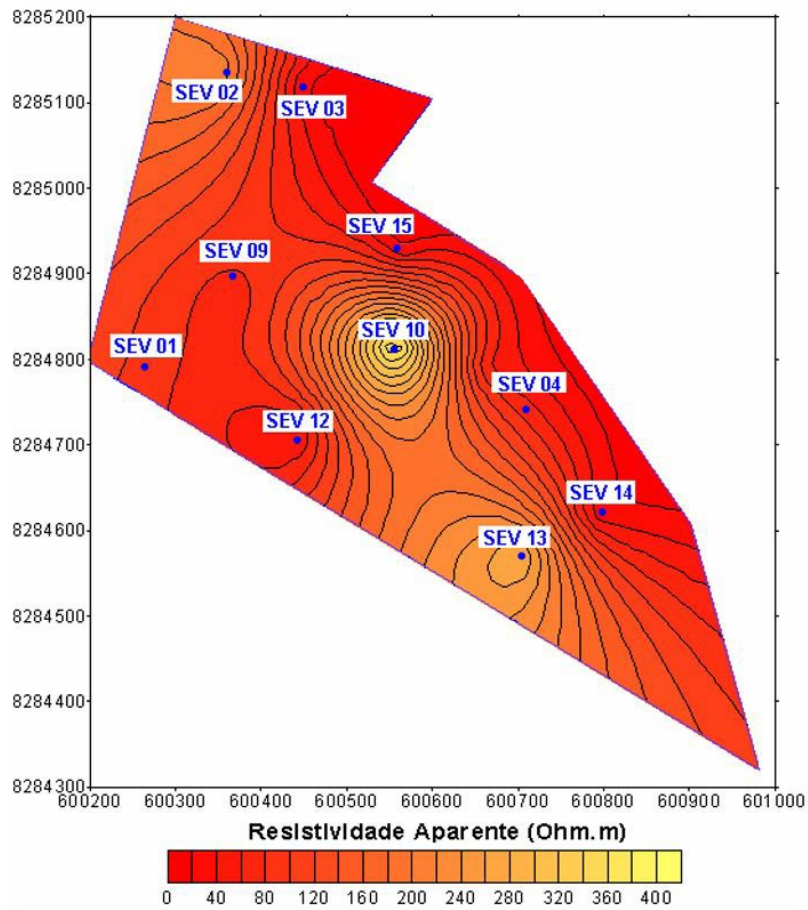
Figura 24 – Mapa de resistividade para a cota 275 metros.
