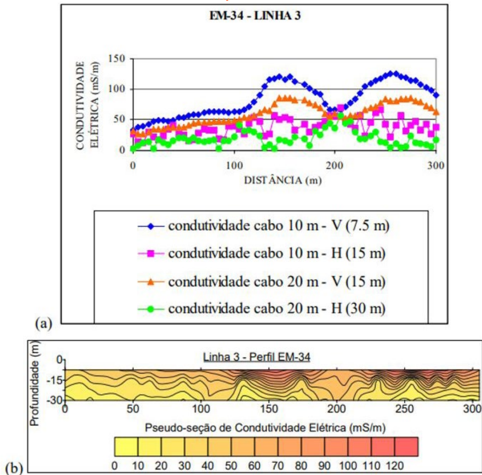
Figura 32 – Perfil de caminhamento eletromagnético da Linha 3 em a) condutividade em função da distância e em b) isovalores da condutividade com a profundidade.
