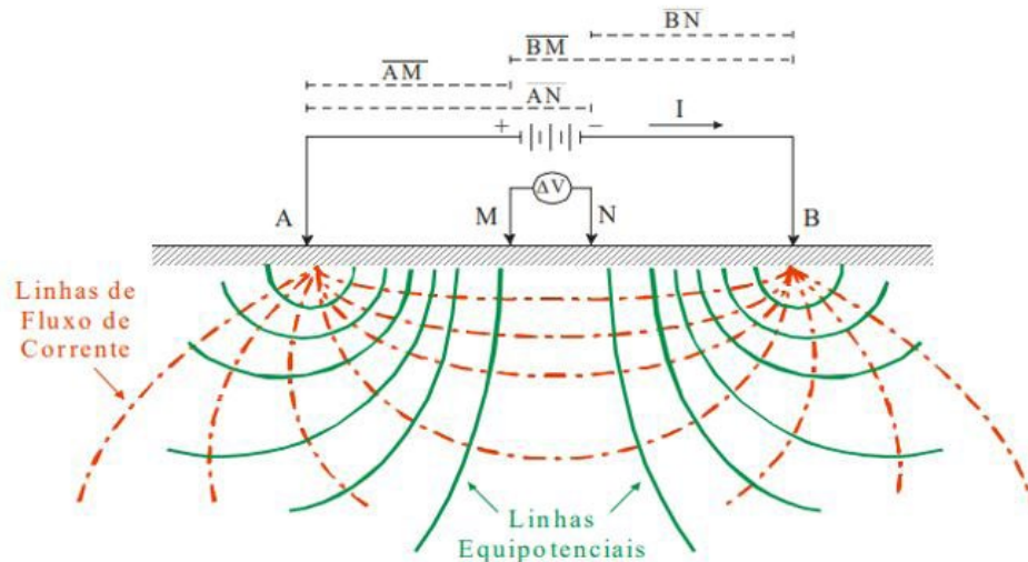
Figura 6 – Distribuição das linhas de fluxo de corrente e das linhas equipotenciais utilizando o arranjo Schlumberger (BORGES, 2002).
