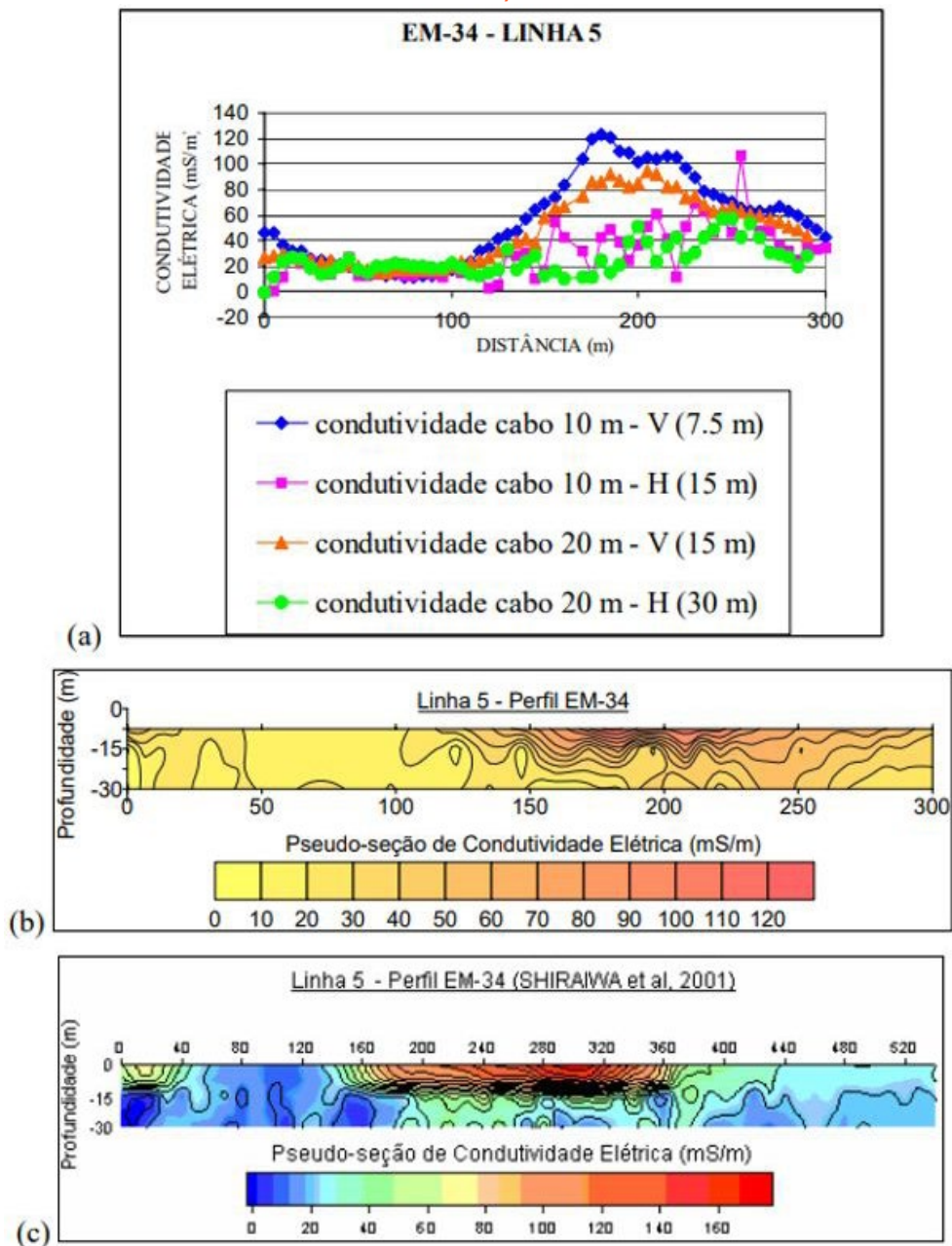
Figura 34 – Perfil de caminhamento eletromagnético da Linha 5 em a) condutividade em função da distância e em b) isovalores da condutividade com a profundidade e em c) isovalores da condutividade (SHIRAIWA et al, 2001).
