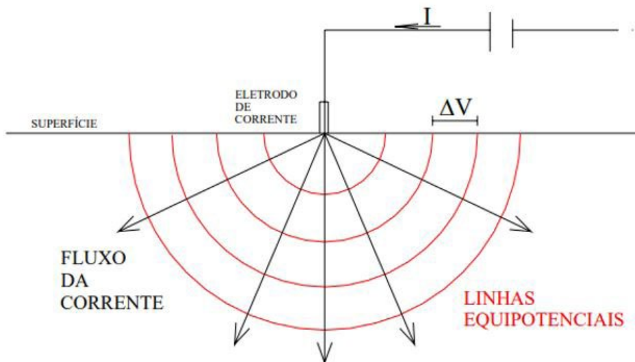
Figura 5 – Representação bidimensional da semi-esfera equipotencial (adaptado de BRAGA, 2002).
