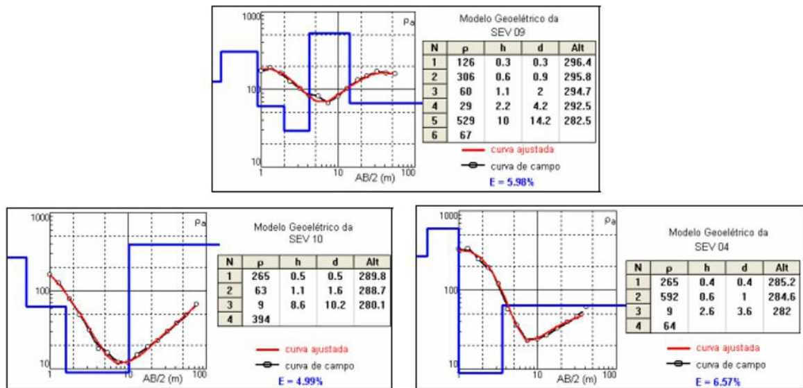
Figura 16 - Modelo geoeletrico das SEVs 04, 09 e 10.
