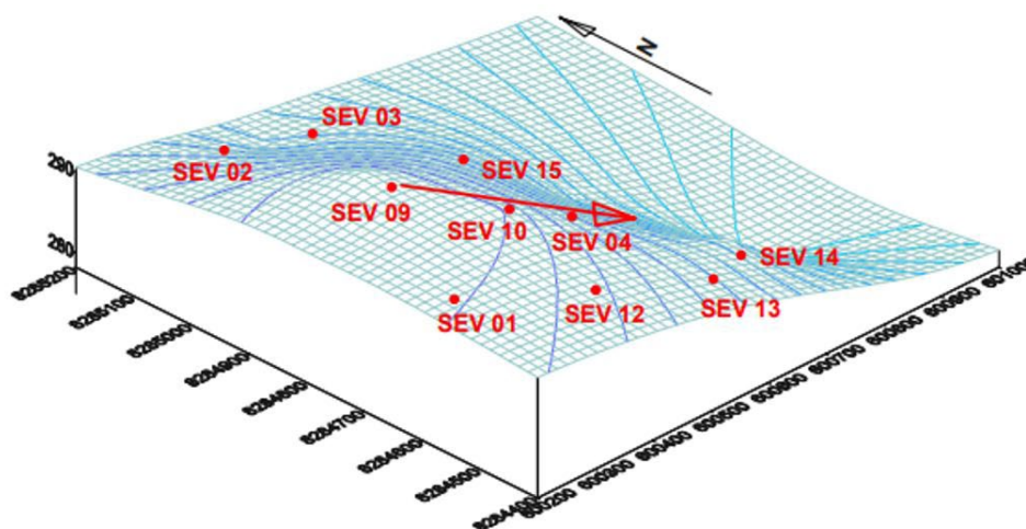
Figura 19 – Mapa potenciométrico do antigo depósito de resíduos.
