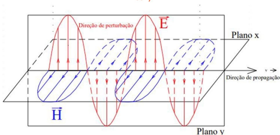
Figura 7 – Propagação da onda eletromagnética (adaptado de REYNOLDS, 1997).
