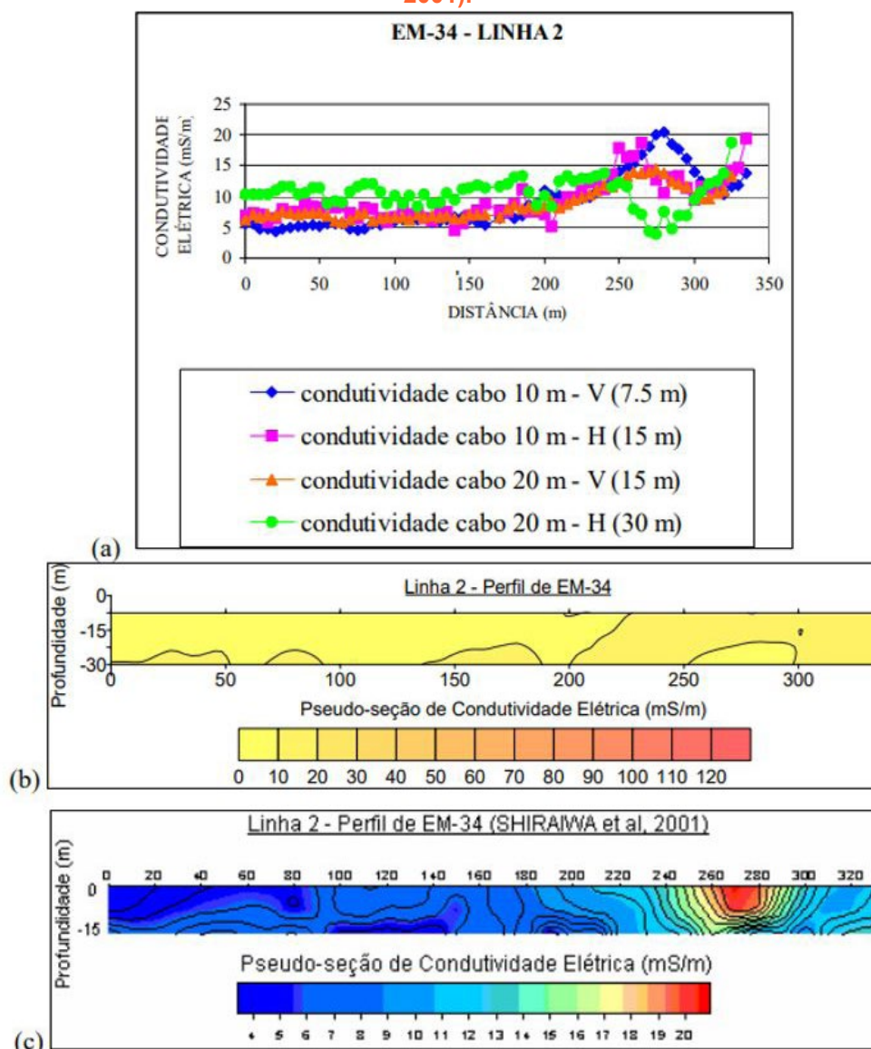
Figura 31 – Perfil de caminhamento eletromagnético da Linha 2 em a) condutividade em função da distância e em b) isovalores da condutividade com a profundidade e em c) isovalores da condutividade (SHIRAIWA et al, 2001).
