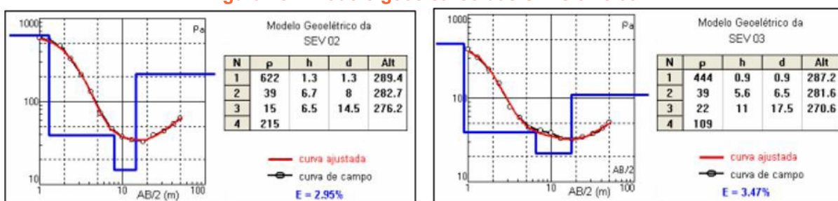
Figura 15 – Modelo geoeétrico das SEVs 02 e 03.
