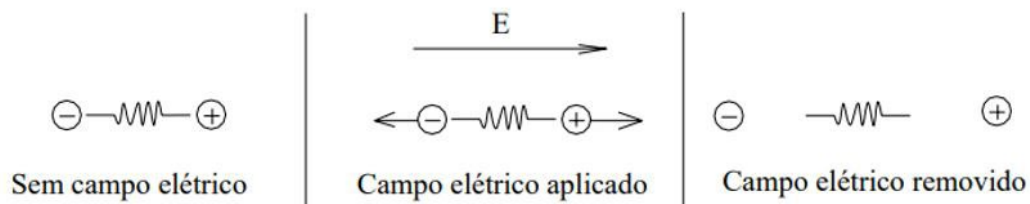
Figura 9 – Movimentação de cargas associada à corrente de deslocamento (adaptado de ANNAN, 1992).
