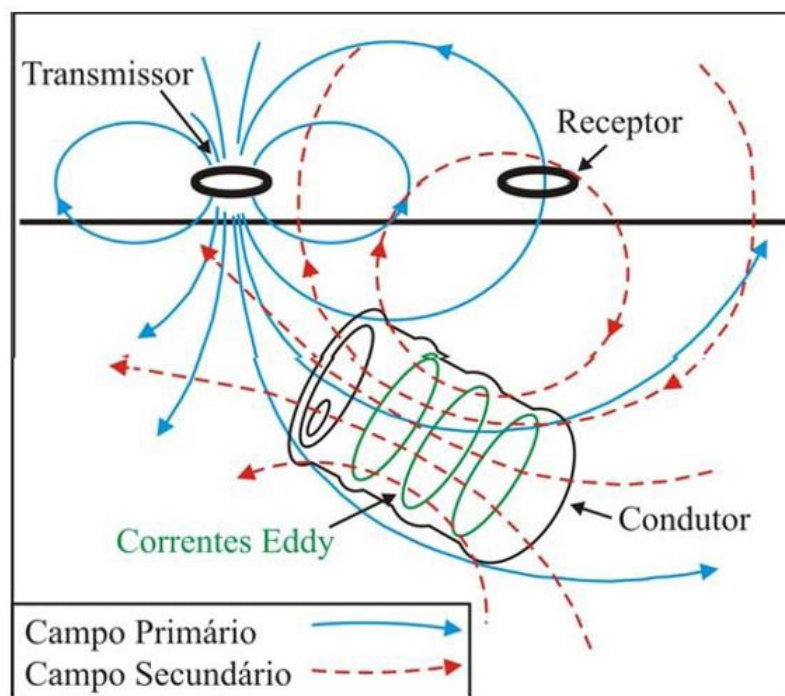
Figura 10 – Indução eletromagnética (adaptado de TELFORD et al, 1990).
