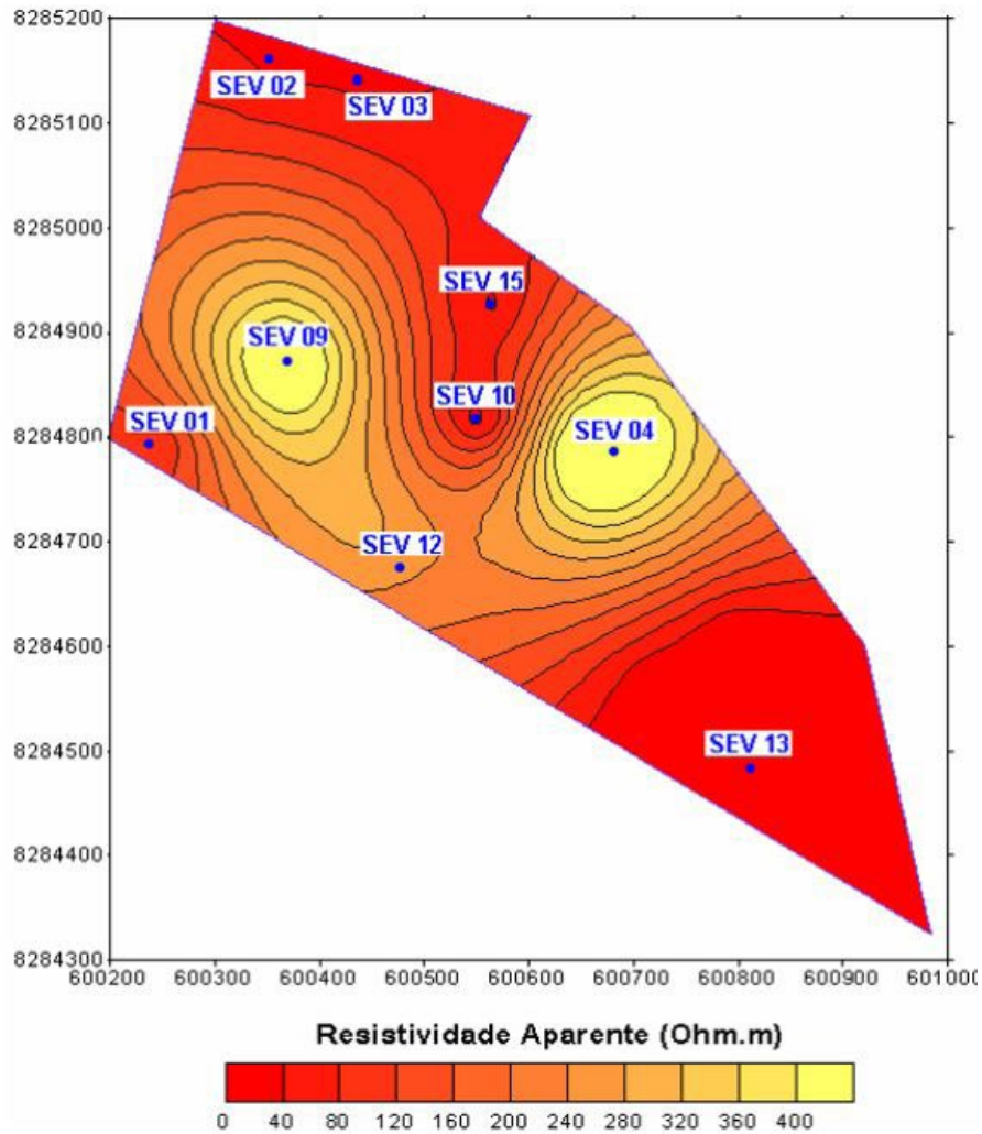
Figura 21 – Mapa de resistividade para a cota 285 metros.
