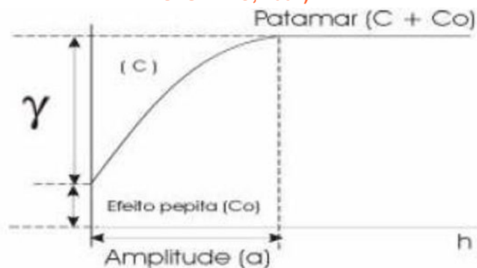
Figura 12 – Semivariograma Usado na Krigagem Ordinária (LANDIM; STURARO, 2002).
