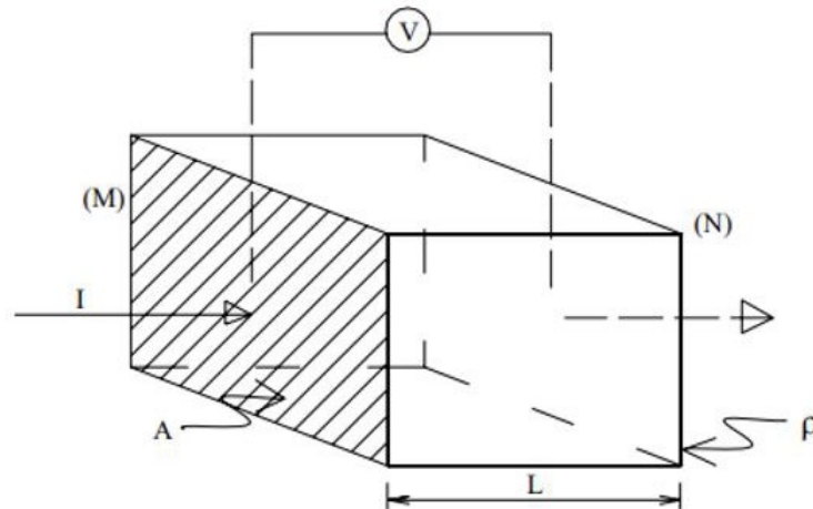
Figura 3 – Bloco homogêneo de definição da resistividade (REYNOLDS, 1997).
