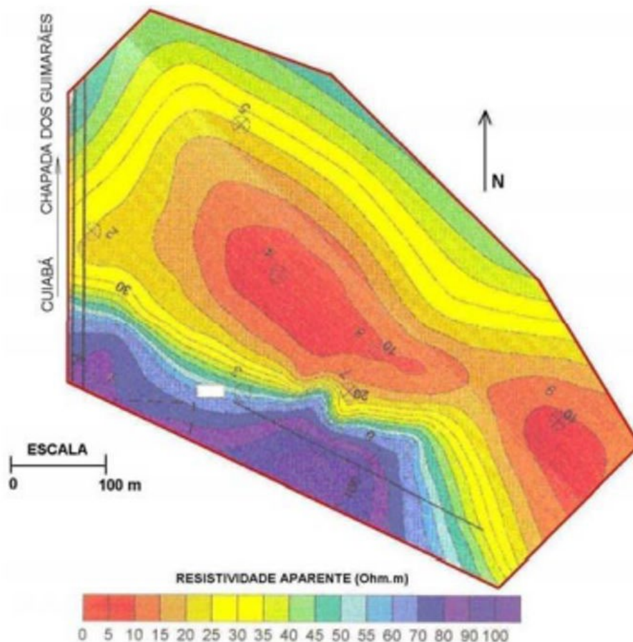
Figura 40 - Mapa de resistividade aparente (ELIS; MATOS, 1995).
