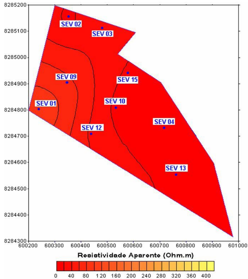
Figura 22 – Mapa de resistividade para a cota 282 metros.
