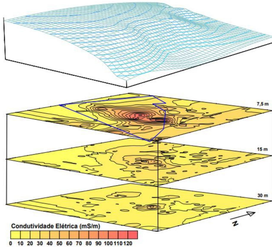
Figura 38 – Mapa de topografia da área e pseudo-seções de condutividade elétrica nas profundidades de 7,5 metros, 15 metros e 30 metros.
