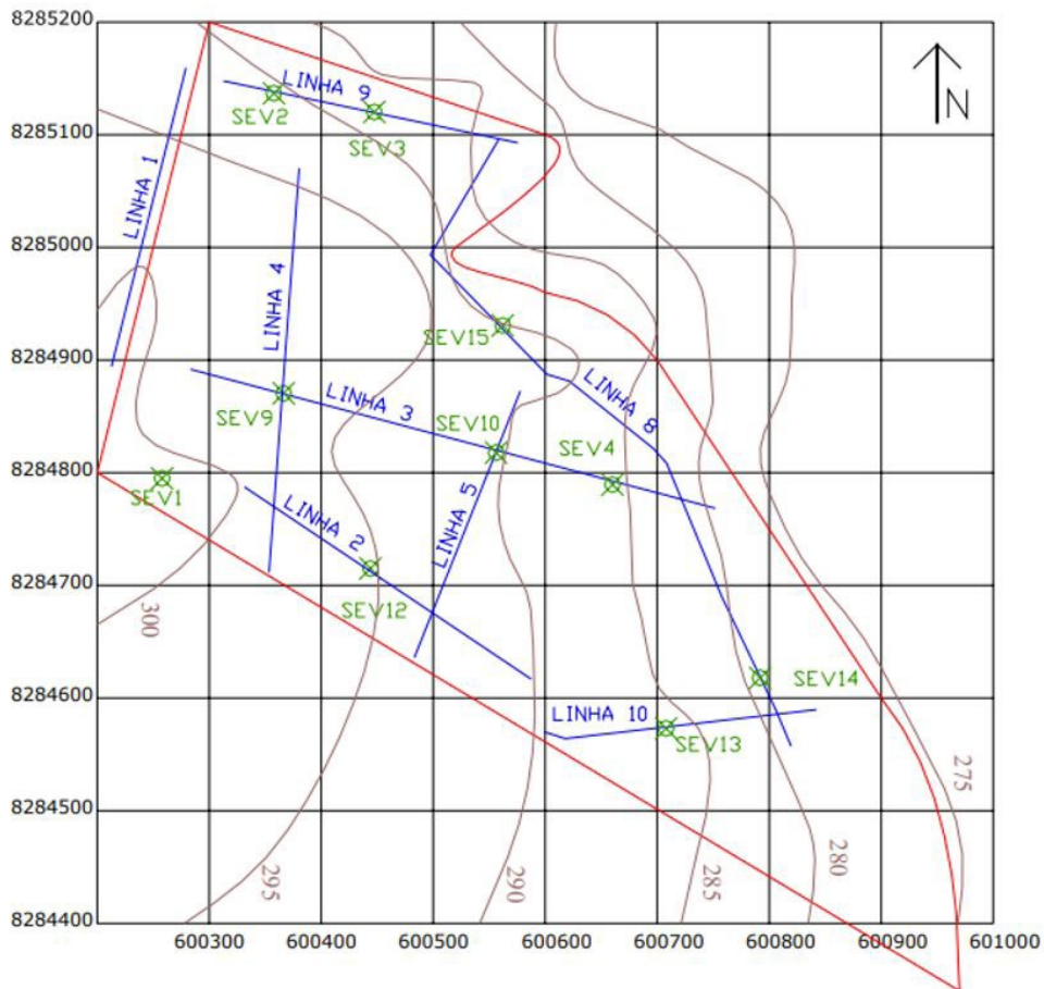
Figura 2 – Localização dos ensaios geofísicos no depósito de resíduos de Cuiabá (SHIRAIWA et al. , 2001).
