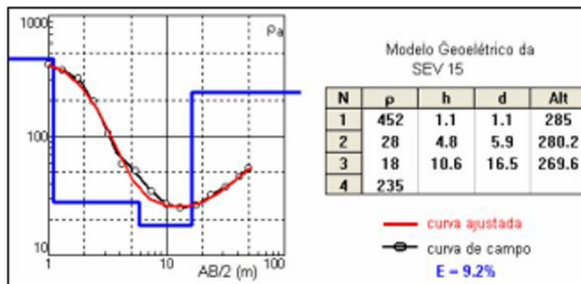
Figura 18 – Modelo geoeétrico da SEV 15.
