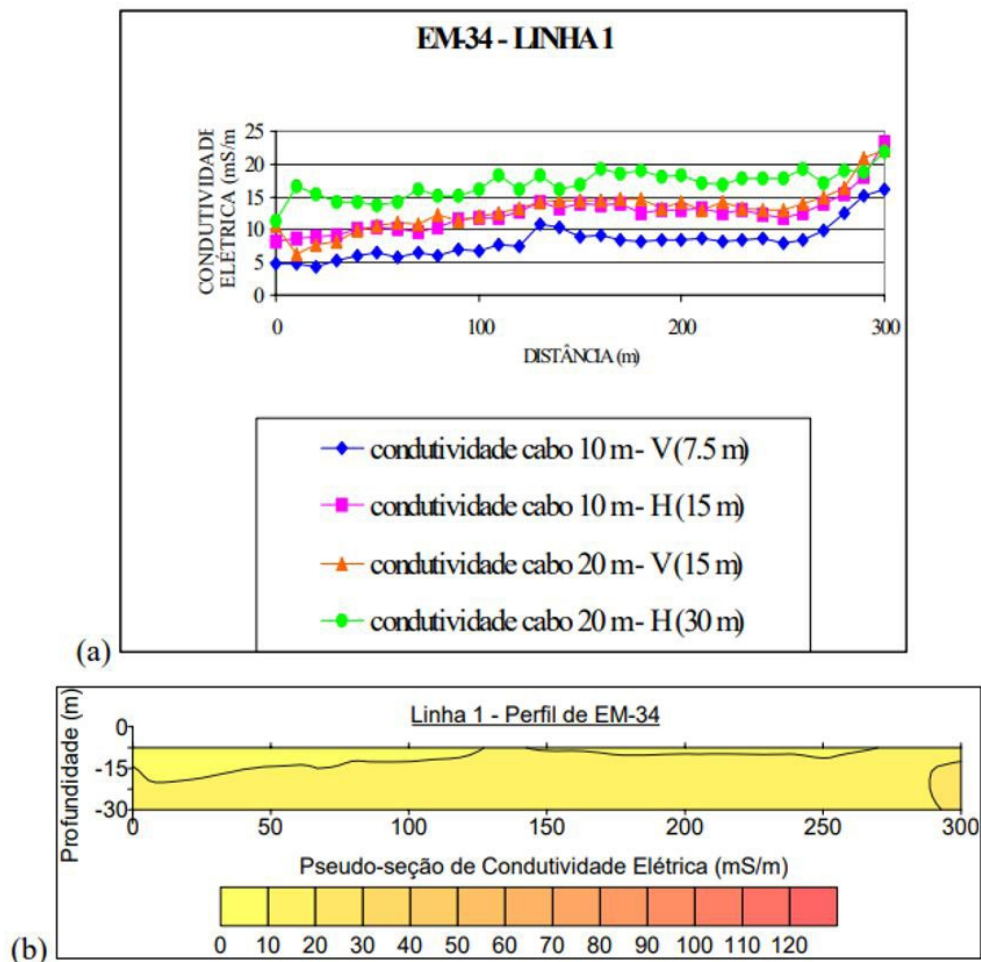
Figura 30 – Perfil de caminhamento eletromagnético da Linha 1 em a) condutividade em função da distância e em b) isovalores da condutividade com a profundidade.
